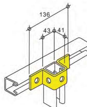
LH1047 - weight 358g
