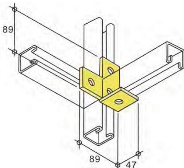
LH1034 - weight 342g
