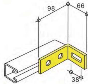
LH1747 - weight 263g
