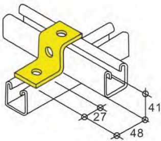
LH1045 - weight 212g
