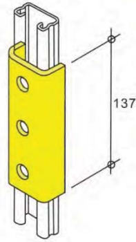
LH4376-A - weight 558g
